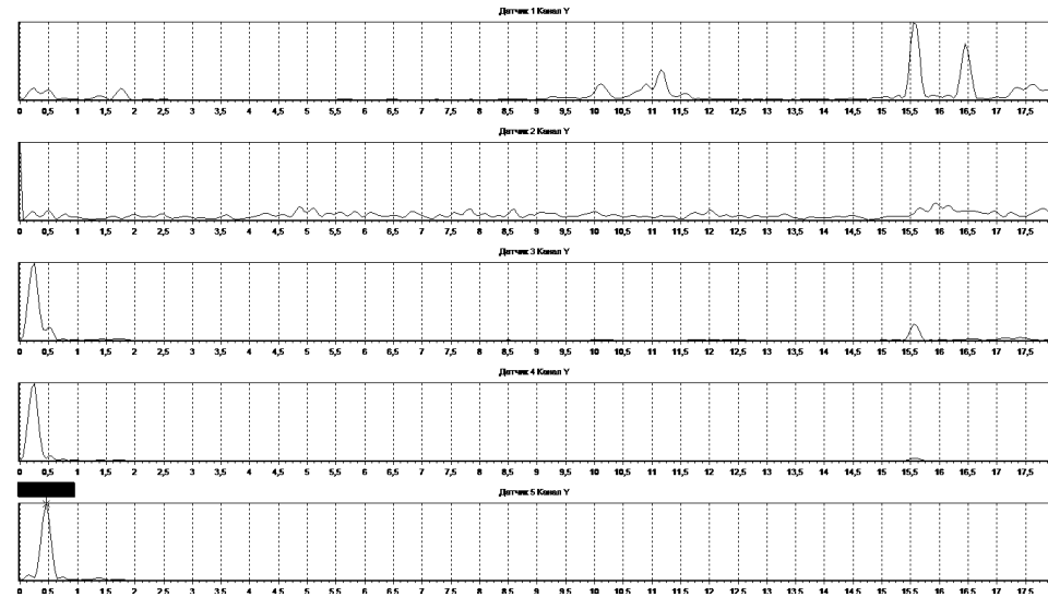
Рис 2.4 Пример спектра колебаний башни по оси Y
