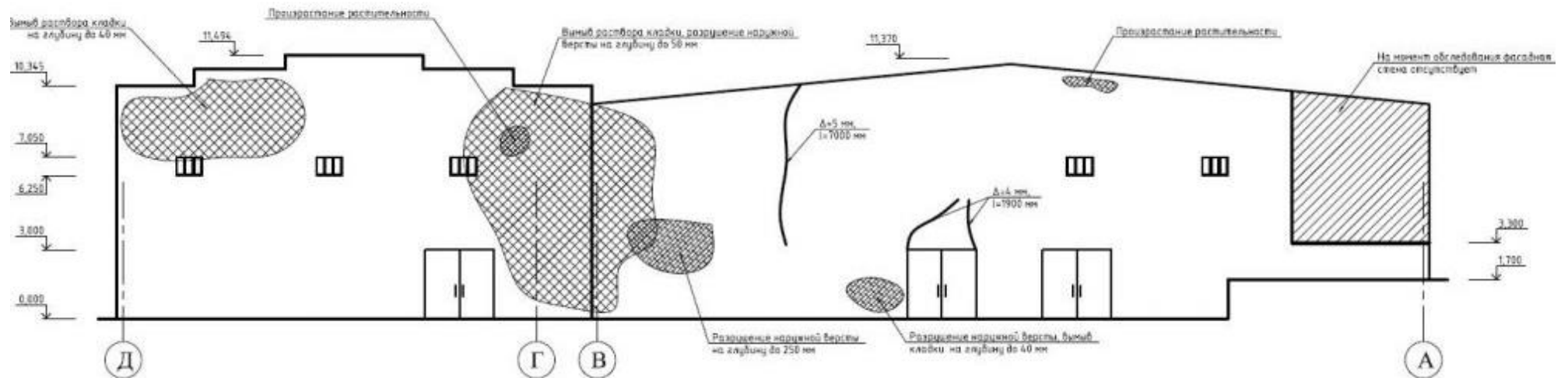
Рисунок 2.1. Пример схемы расположения дефектов на фасаде здания
