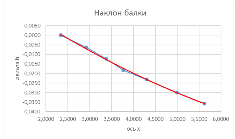
Рис. 2.4. Пример изображения расчетного уклона балки
