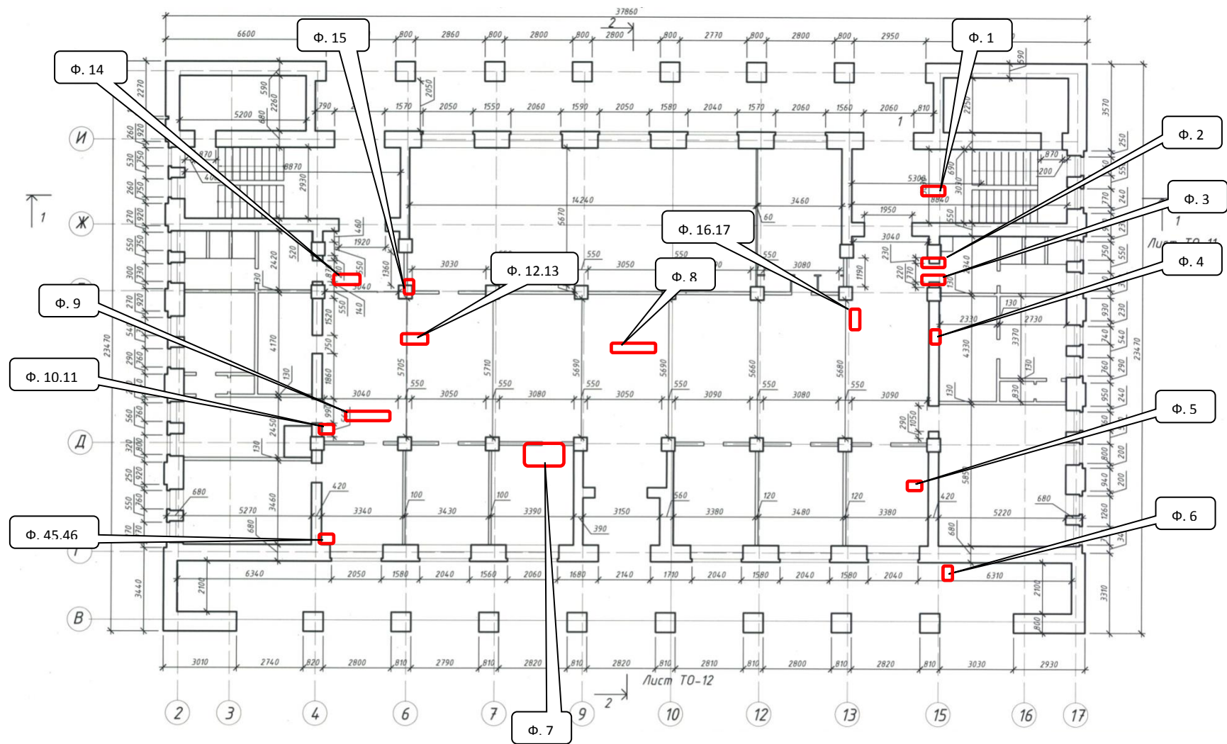
Рисунок 2.2. Пример схемы расположения дефектов в плане
