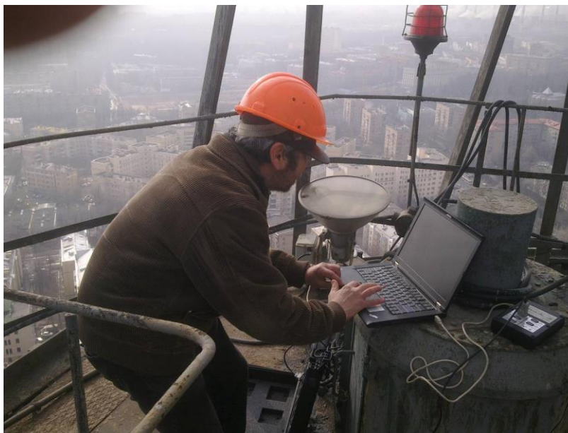
Рис. 2.2. Пример оборудования пункта сбора динамических данных на верхней площадке стальной башни
