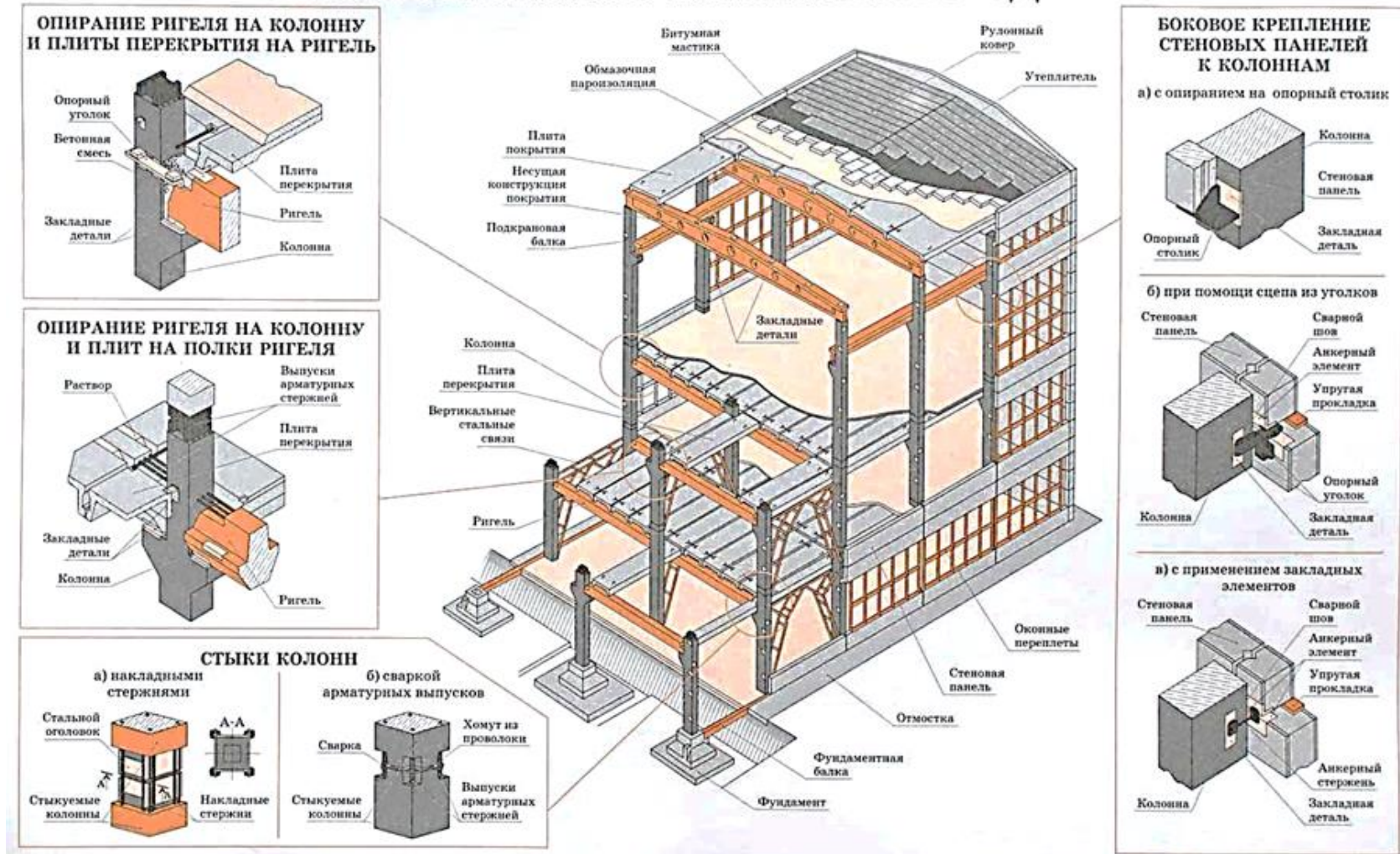
Рисунок 2.5. Основные конструктивные элементы многоэтажного промышленного здания
