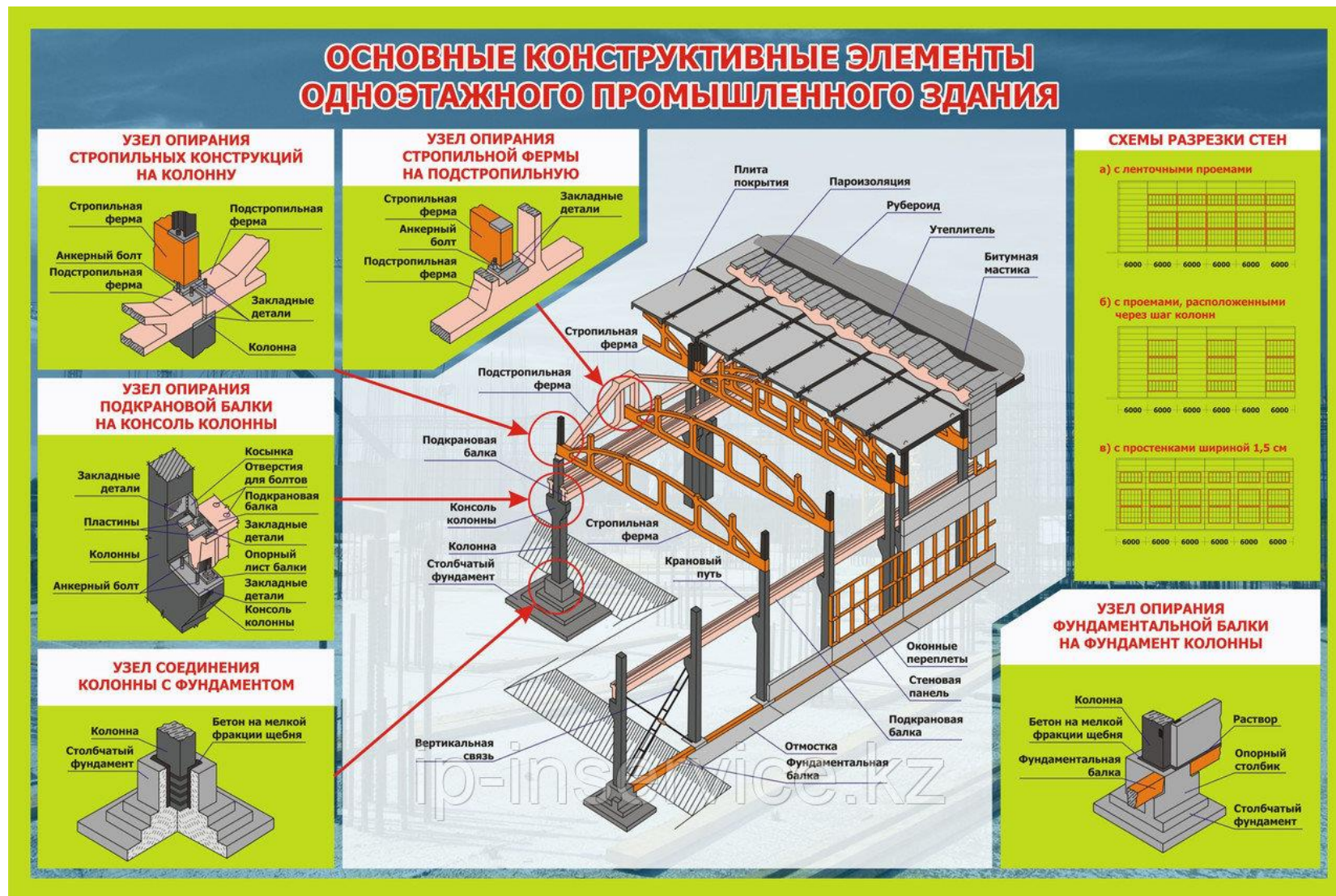
Рисунок 2.4. Основные конструктивные элементы одноэтажного промышленного здания
