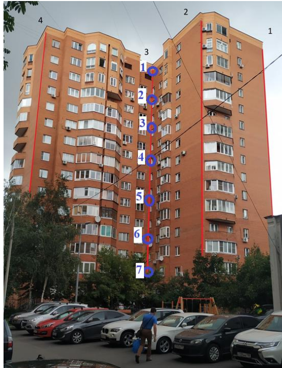
Рис. 2.1. Геодезические измерения снаружи здания (красными линиями показаны оси измерения, а синими кружками – точки измерений)
