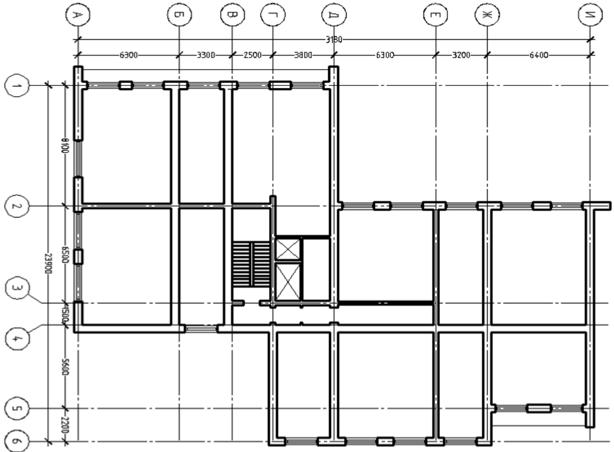
Рисунок 2 – Пример плана типового этажа здания
