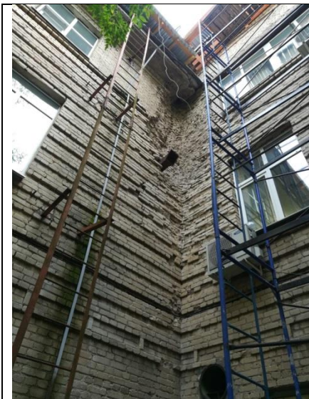
Фото 5. Место разрушения кирпичной кладки в месте сопряжения кирпичных наружных несущих стен здания в осях К-Л/14-15
